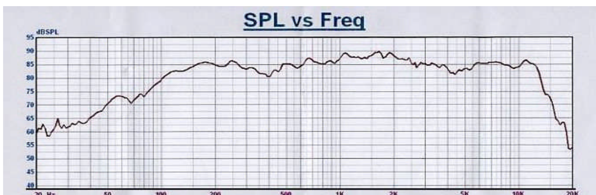
MP100FL25FE-43C 10 cm フルレンジ UNIT 周波数特性 ( JIS 規格箱測定 )
